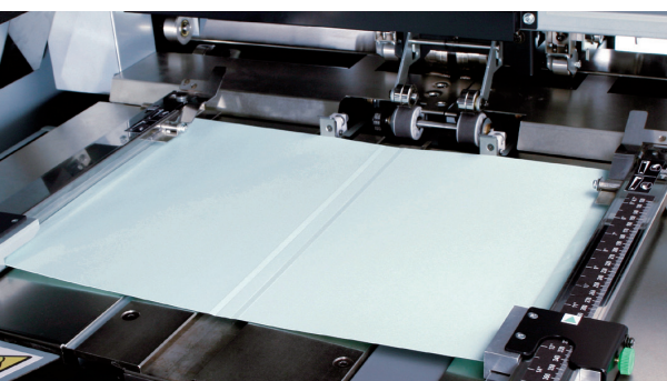
Omslagen worden automatisch gerild en op de kneep tafel gelegd
