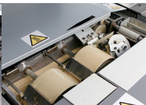
Lijmtrommels met automatische zij-belijming
